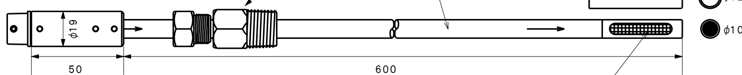
(b) プローブ概観図
